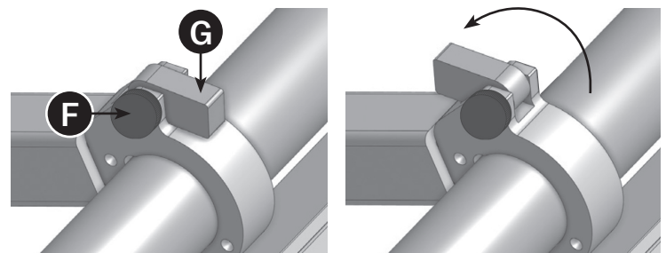
ANTIRRETROCESO ABAJO
